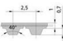
Passo T 2,5
